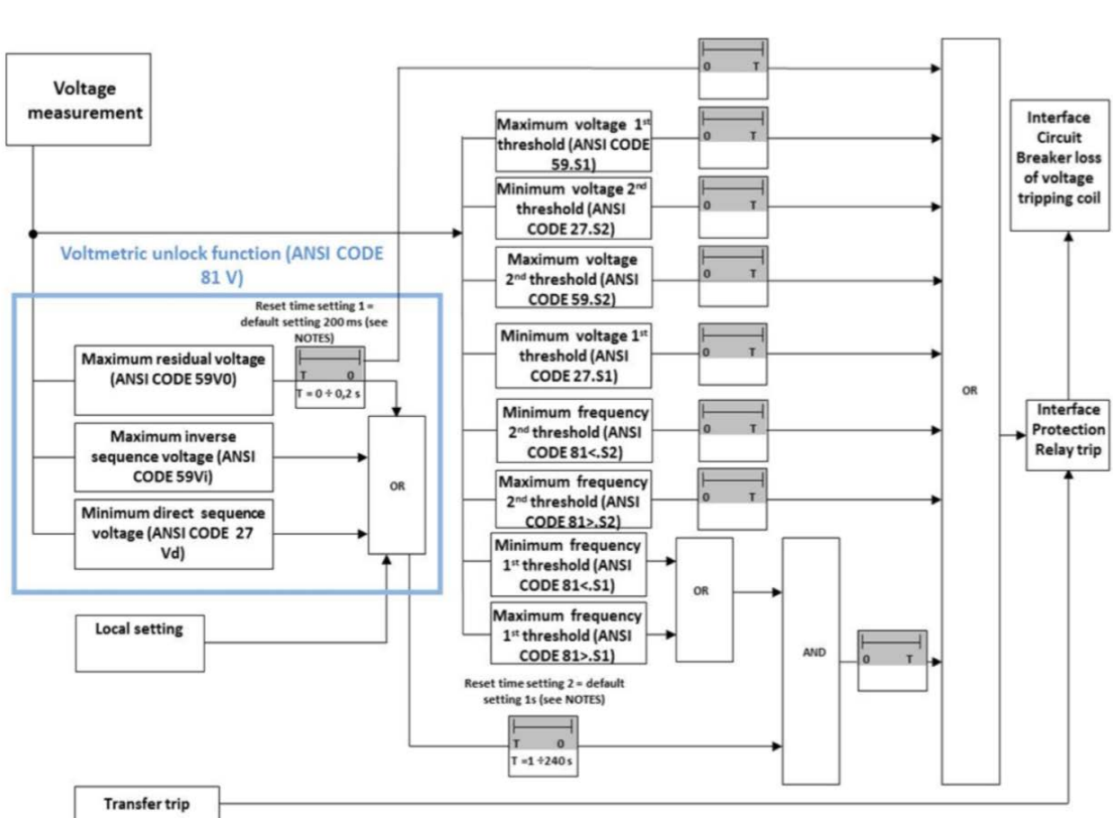
Figure 7 - Schéma de principe pour une protection de détection d'îlotage avec l'activation d'une fenêtre de fréquence plus fine sur base de critères locaux de la tension (source: EN50549-1 :2019 et EN50549-2 :2019)
