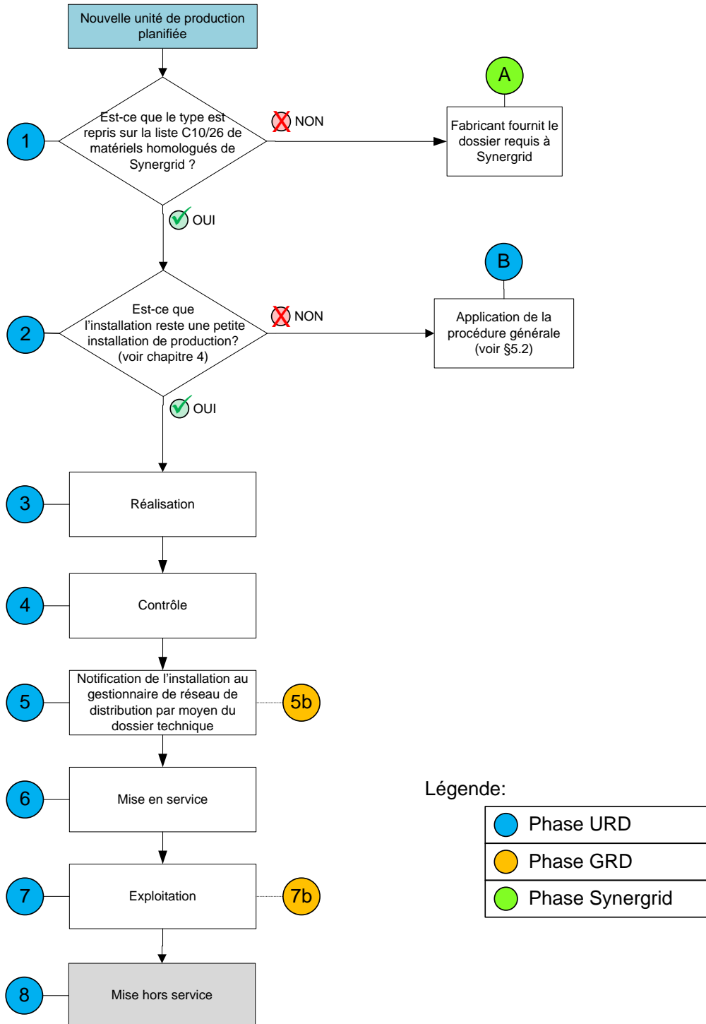
Figure 4 - Procédure simplifiée de mise en service d'une petite installation de production d'électricité
